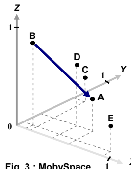
Fig. 3 : MobySpace
